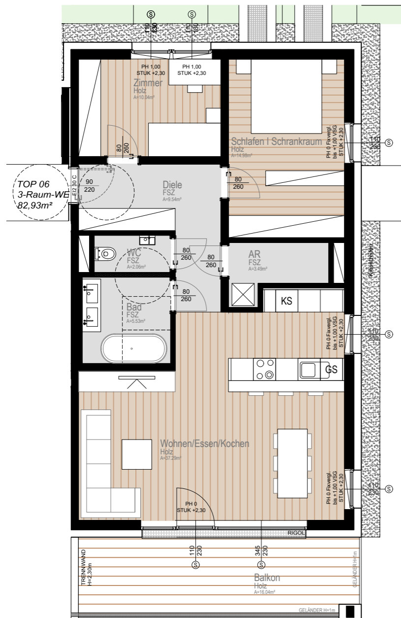
ERDGESCHOSS | TOP 06 M 1:100
