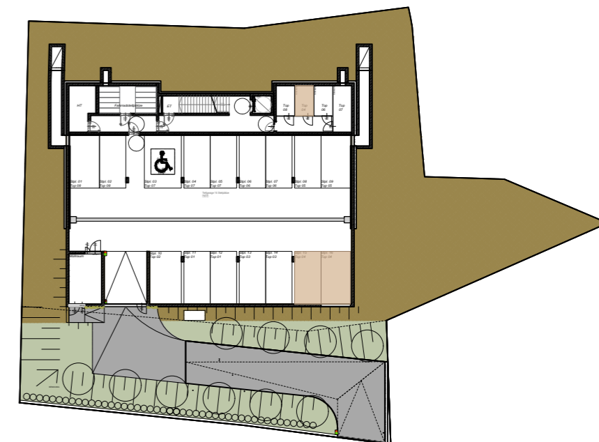
KELLERABTEIL I TIEFGARAGENSTELLPLÄTZE M 1:500
