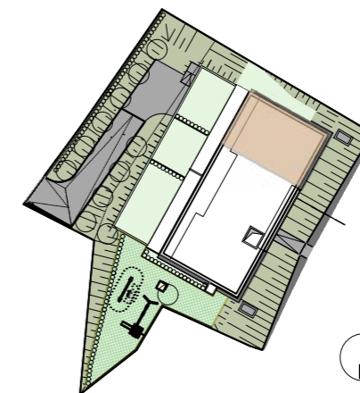
LAGEPLAN M 1:1000
