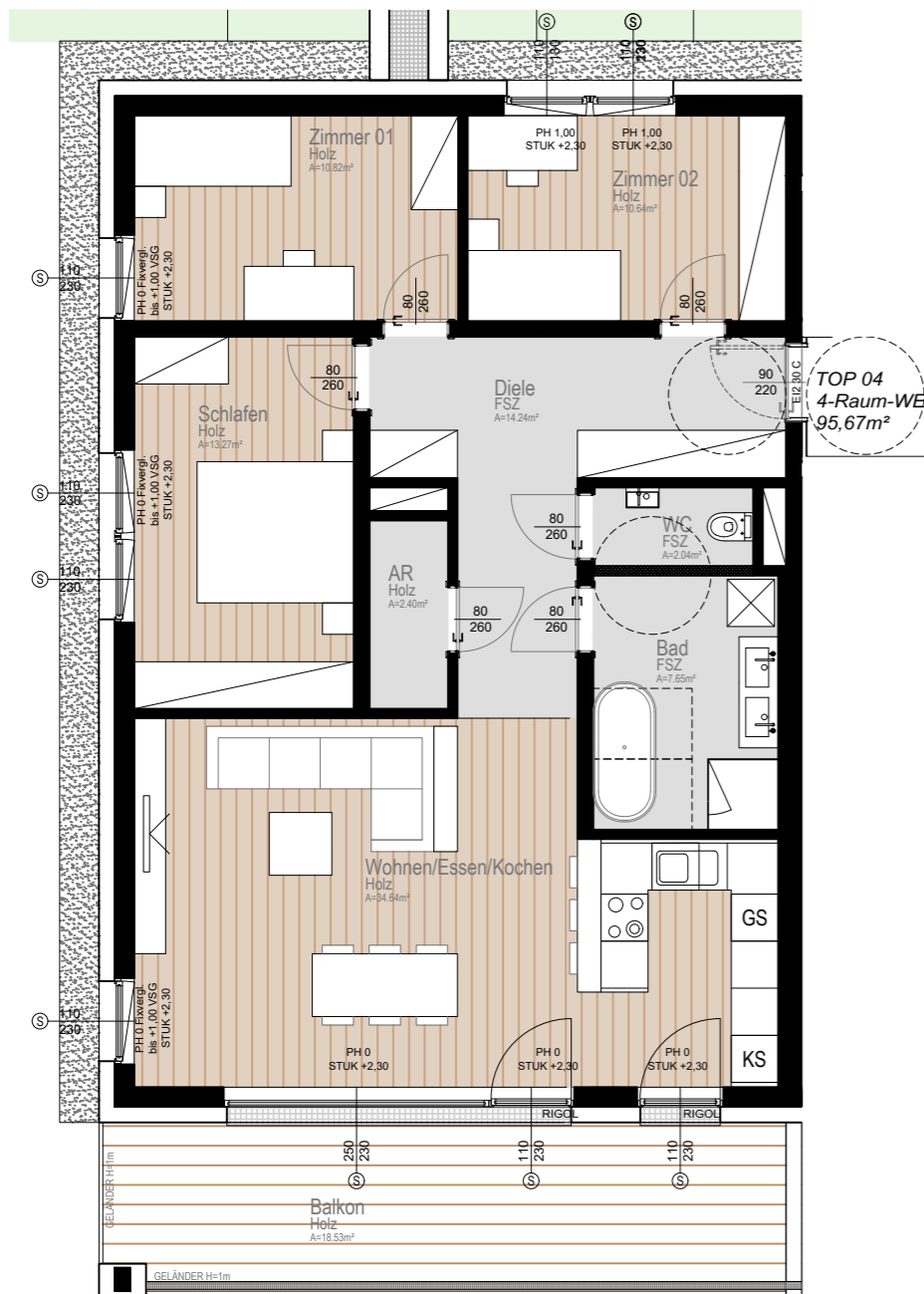
ERDGESCHOSS I TOP 04 M 1:100
