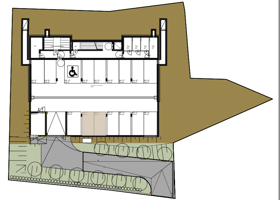
TIEFGARAGENSTELLPLÄTZE M 1:500
